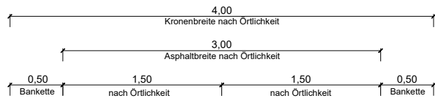
Regelquerschnitt ab Bau-km 0+827
