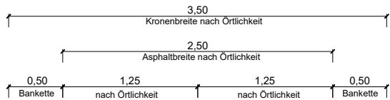
Regelquerschnitt Radweg Asphaltbreite: 2,50 m
