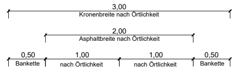
Regelquerschnitt Radweg Asphaltbreite: 2,00 m
